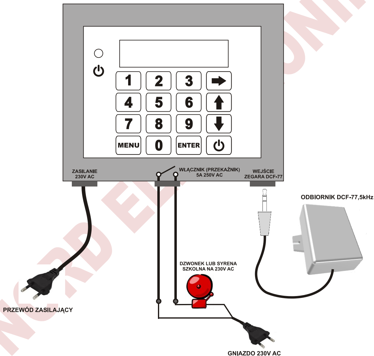
Rysunek 1. Podłączenie urządzenia
